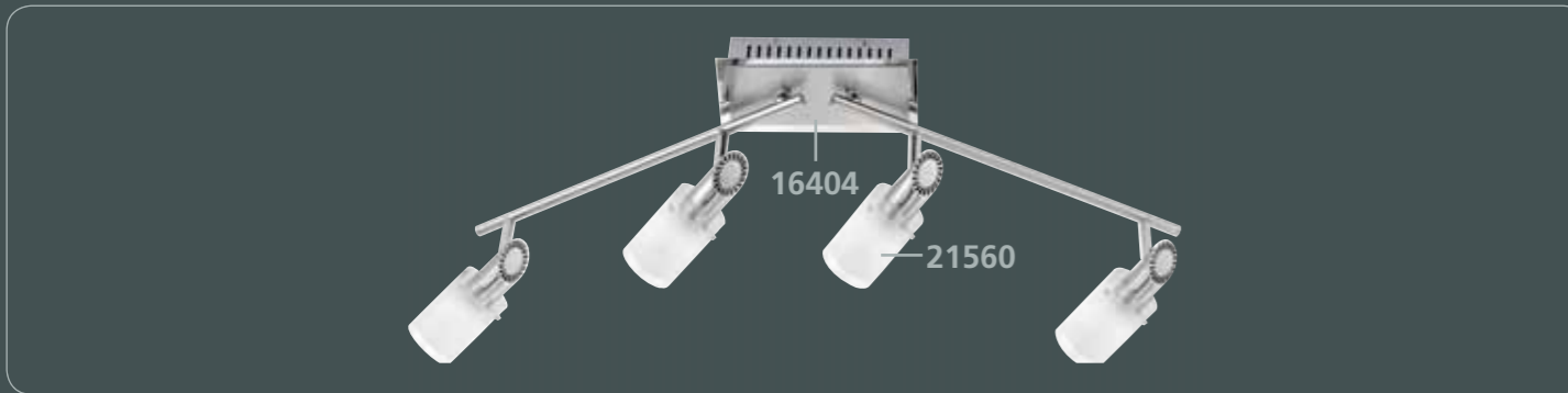
Nickel matt/chrom · Nickel matt/chromium · 86 cm x 10 cm · ↳ 16 cm incl. 4 x LED 4,2 W / 3000 K / 4 x 477 lm
